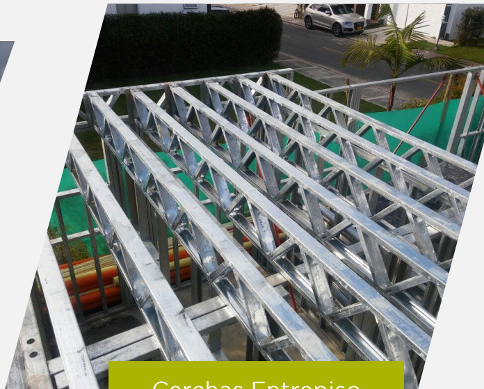
Cerchas Entrepiso
