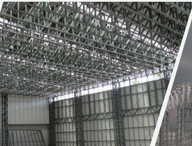
Muros interiores y cerchas
